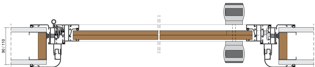
PORTA CON ANTA INTELAIATA CON FASCIA CON IMBOTTE 1 / FRAMED DOOR WITH INFILL PANEL AND JAMB 1
