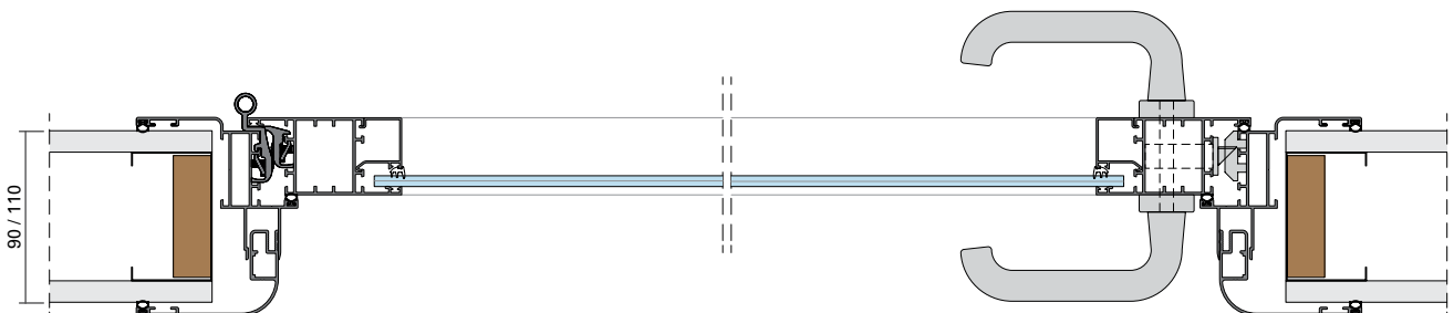
PORTA VETRATA CON ANTA INTELAIATA CON IMBOTTE 1 / GLAZED DOOR WITH ALUMINIUM FRAME AND JAMB 1
