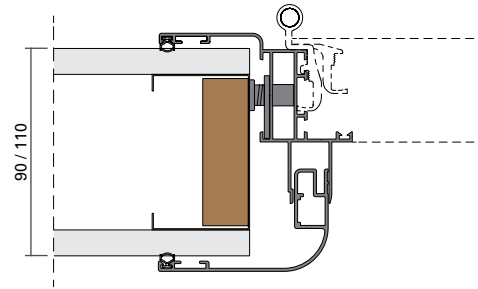
IMBOTTE 1 - spessore 90/110 mm / JOLLY JAMB - thickness 90/110 mm
