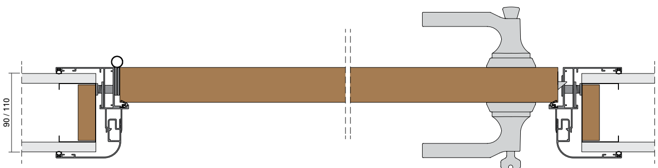
PORTA BATTENTE CIECA TAMBURATA CON IMBOTTE 1 / FRAMELESS HONEYCOMB DOORS WITH JAMB 1
